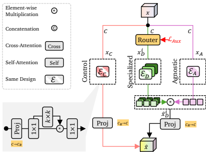
(b) Degradation-aware Learner (DaLe) + Controller (C)
